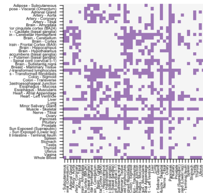
(b) GoM thin 0.01
