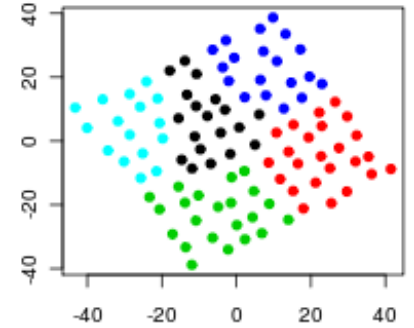
d) K=5
