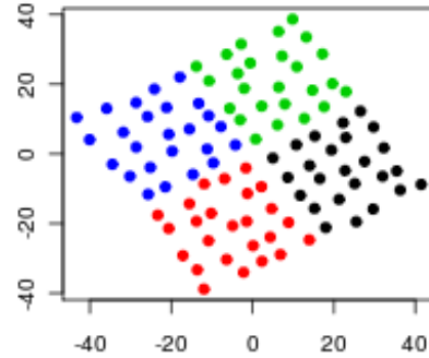
c) K=4
