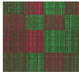
(2) pcNormal36
