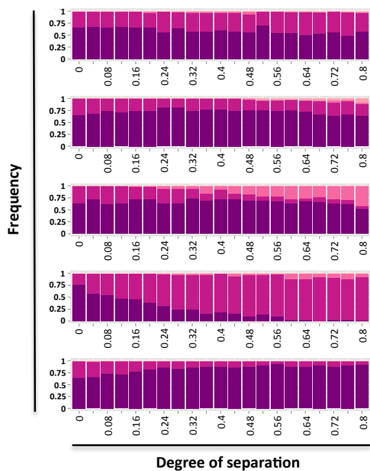
d) GAP-PC
