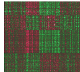
(3) pcNormal39
