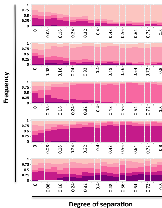
e) Modified GAP-PC
