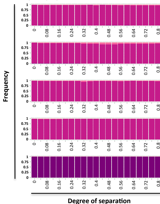
b) \Delta(K)
