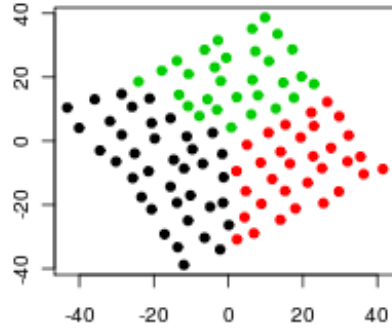
b) K=3
