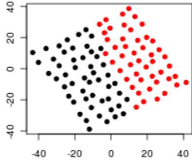
a) K=2
