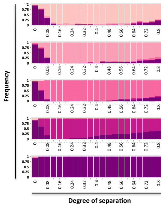
a) PAC
